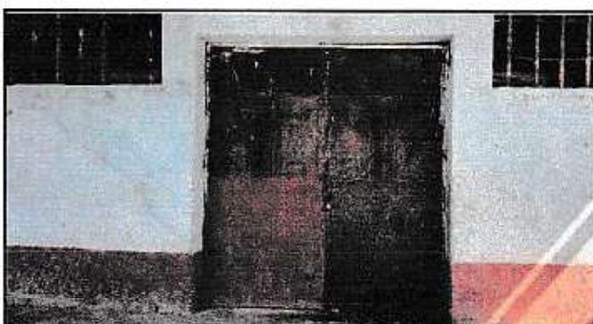
Foto 4: Puerta doble de metal en mal estado, foto de la parte externa. Cada puertas tiene las siguientes medidas: 2 metros de ancho por 2 metros de alto
